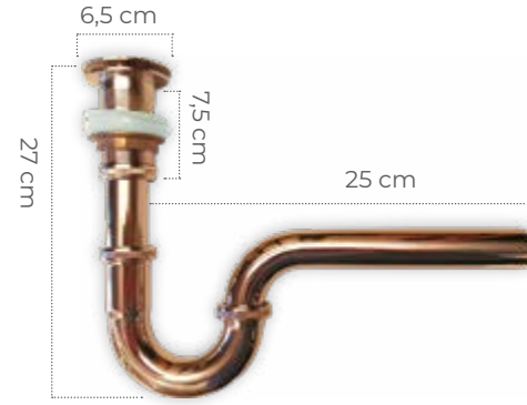
SFN-03 Pop-up “U” Sifon Paslanmaz Bronz
