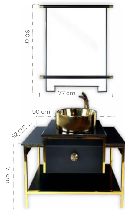
MBU-7300 Gold Metal Alt Ve Üst Banyo Ünitesi 90 cm G-224 Luxury Altın Çanak Lavabo Bataryası
