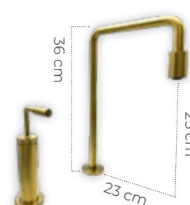
ELG-113 Elite Lüks Gold Lavabo Bataryası
