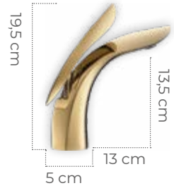
G-223 Luxury Gold Lavabo Bataryası
