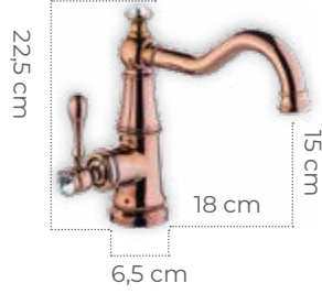
F-238 Eda Bronz Lavabo Bataryası
