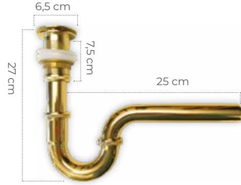
SFN-02 Pop-up “U” Sifon Paslanmaz Altın
